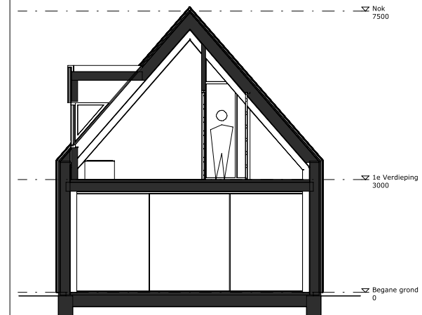
Doorsnede
